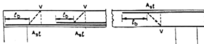
Fig. 3-1 per l_b , lunghezza di ancoraggio, vedasi punto 5.3.3.
